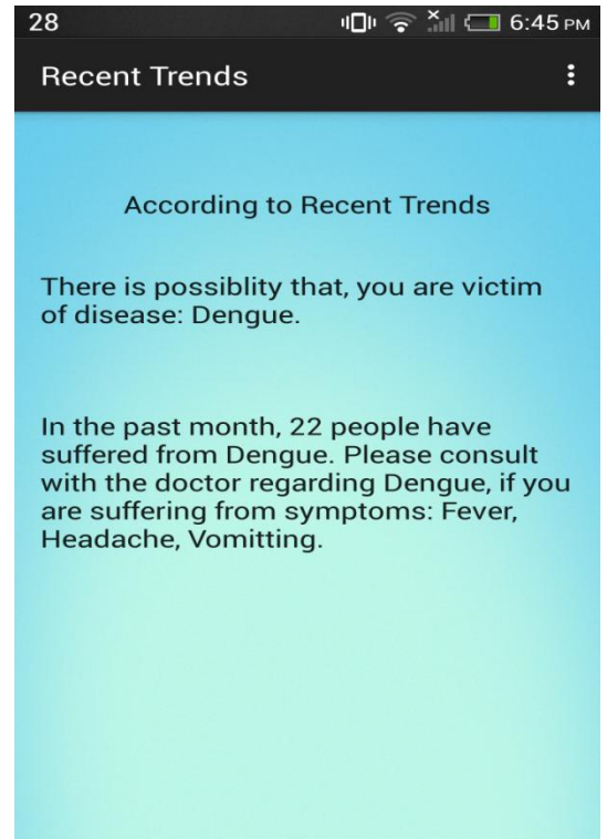
Fig. 7. - Recent Trends
