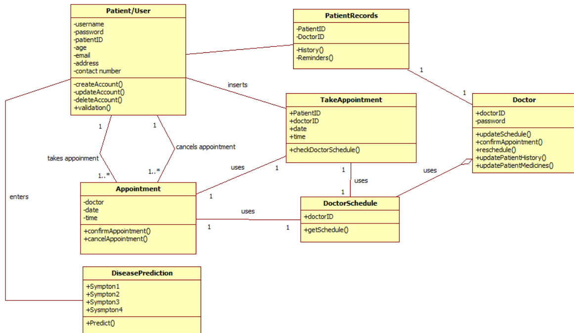
Fig. 4. - Schema
