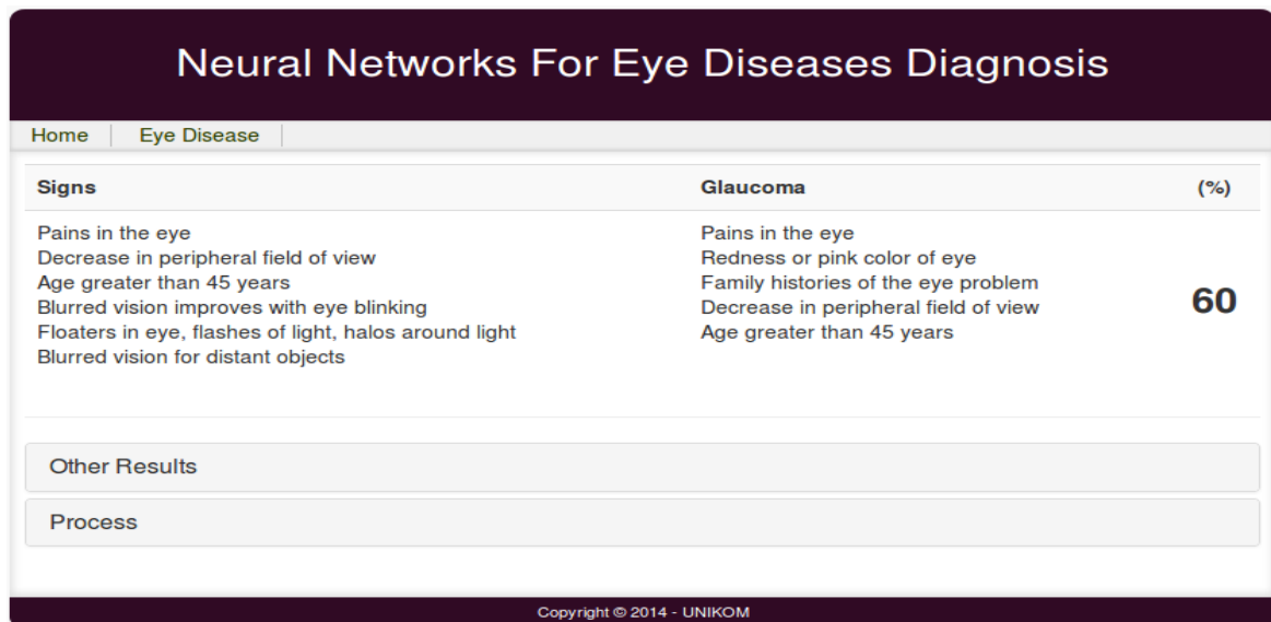
Fig. 2.- Result[3]
