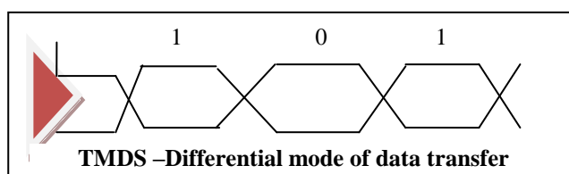
Fig:3 TMDS Protocol
