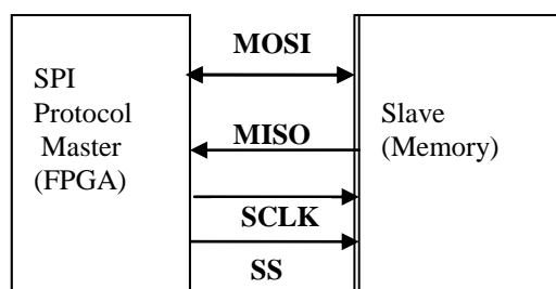
Fig:1 SPI Protocol
